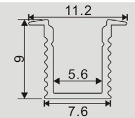
吸顶式安装 Ceiling mount
