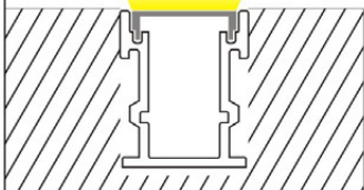
地面嵌入式安装 embedded installation
